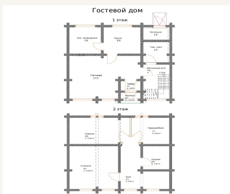
План 1 и 2 этажей
